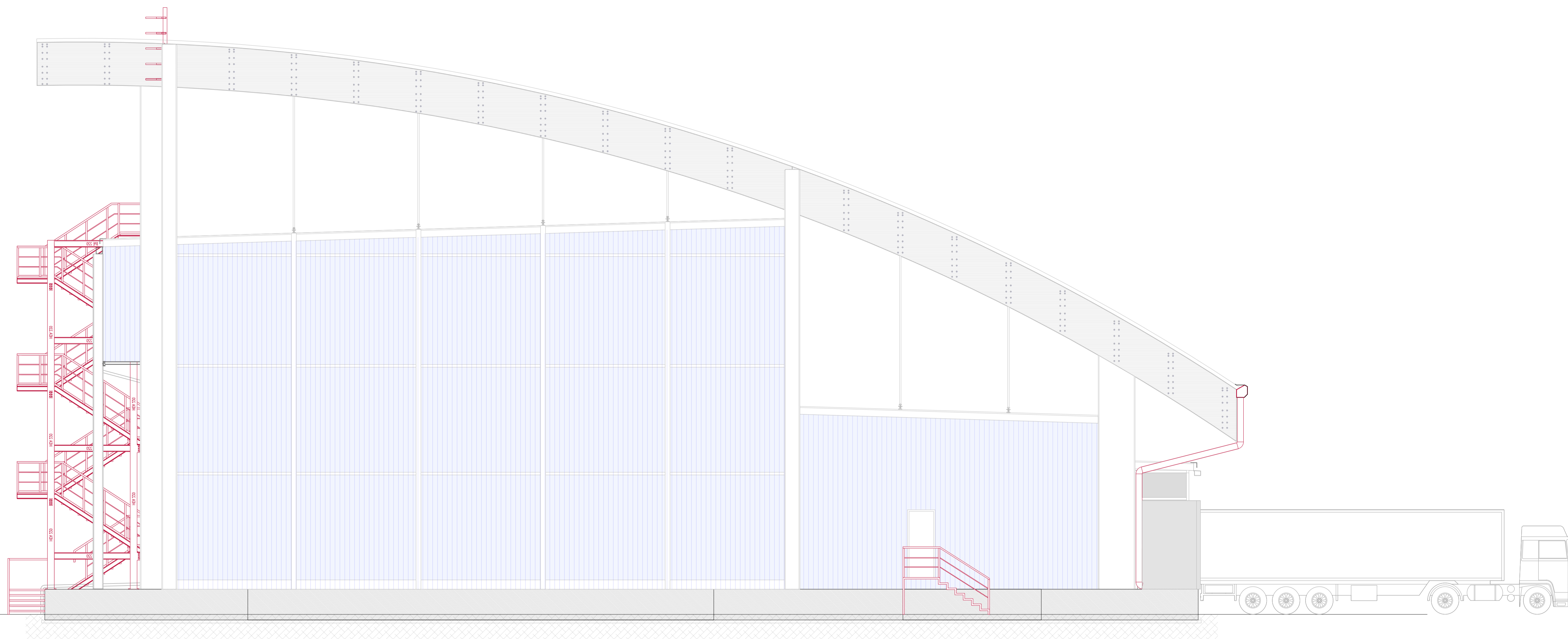
Prospetto Ovest
